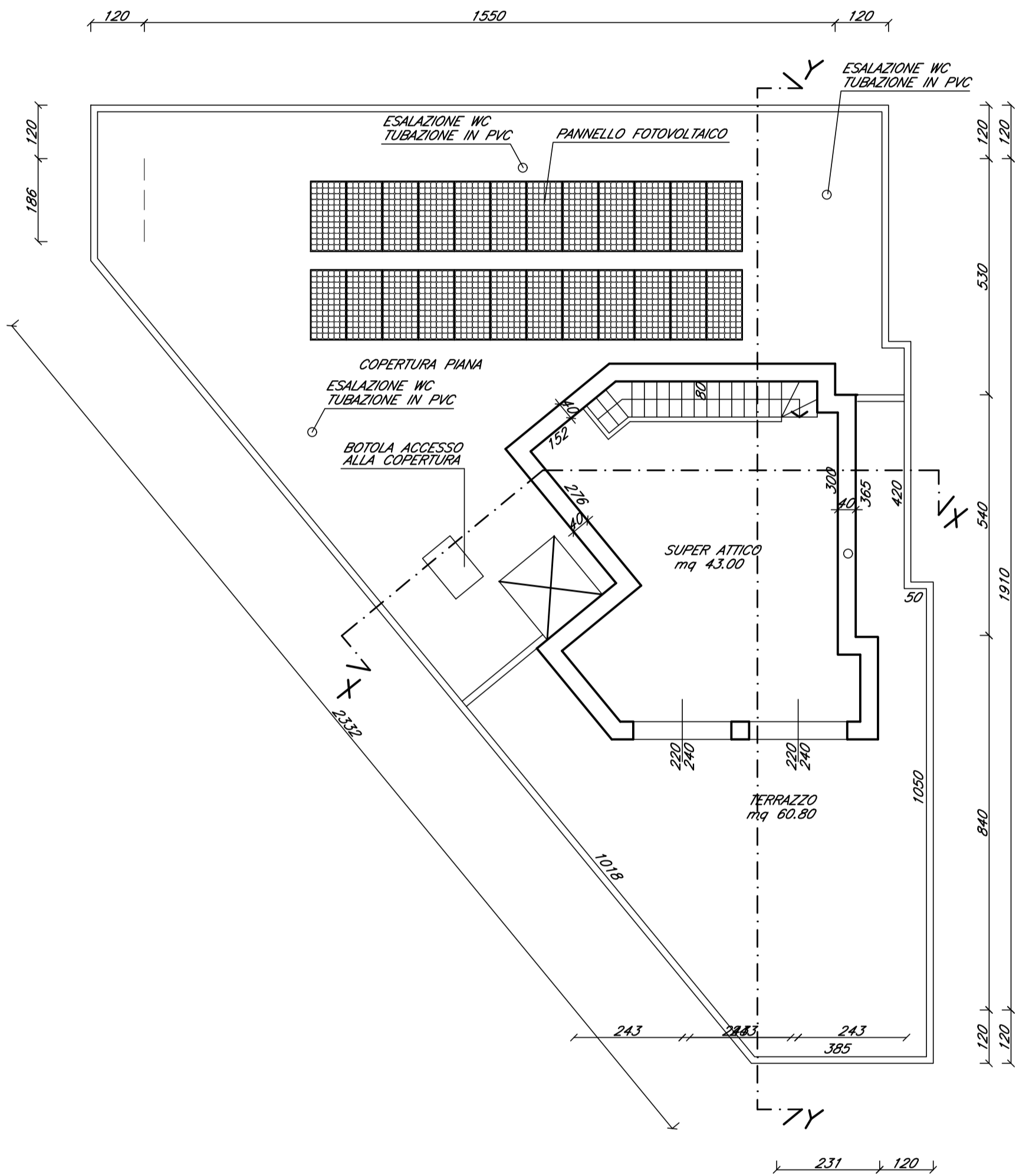
PIANTA PIANO SESTO SCALA 1:100
